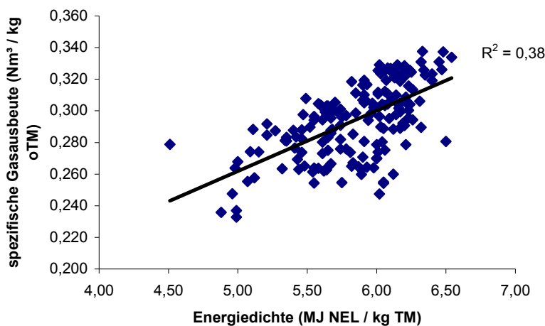
Abbildung 3: spezifische Methanausbeute ( \text{Nm}^3 / \text{kg oTM} ) in Relation zur Energiedichte (MJ NEL / kg TM)
