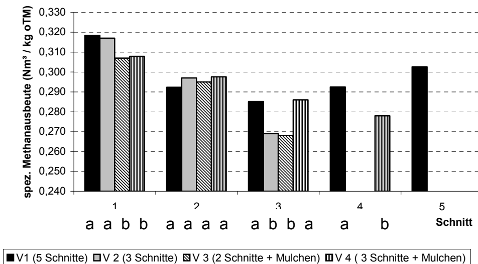
Abbildung 5: Mittlere spezifischen Methanausbeuten in Nm³ / kg oTM der unterschiedlichen Aufwüchse
