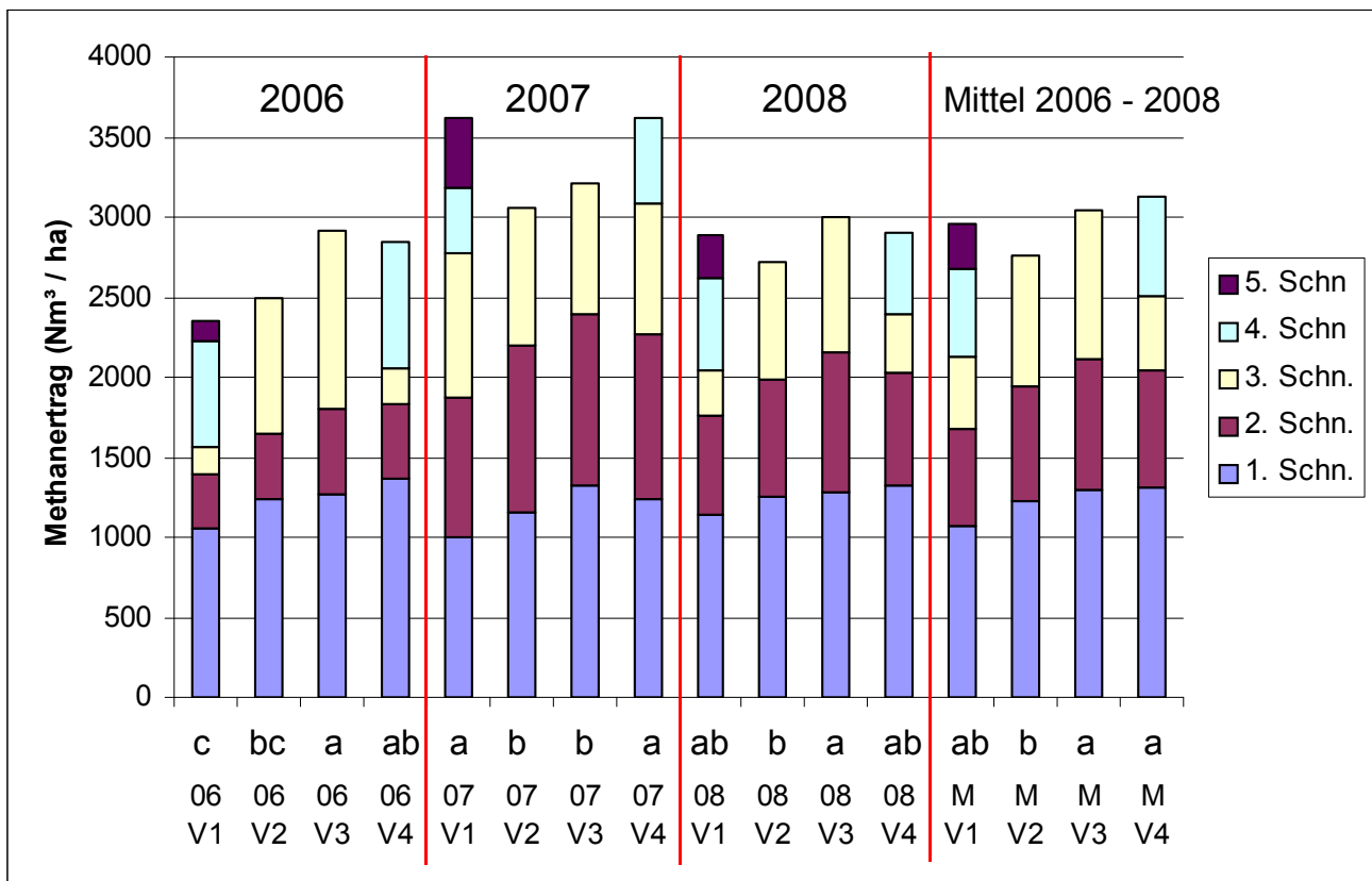
Abbildung 10: Jährlicher Methanertrag in Nm 3 / ha der einzelnen Varianten mit Berücksichtigung der Mulchschnitte
