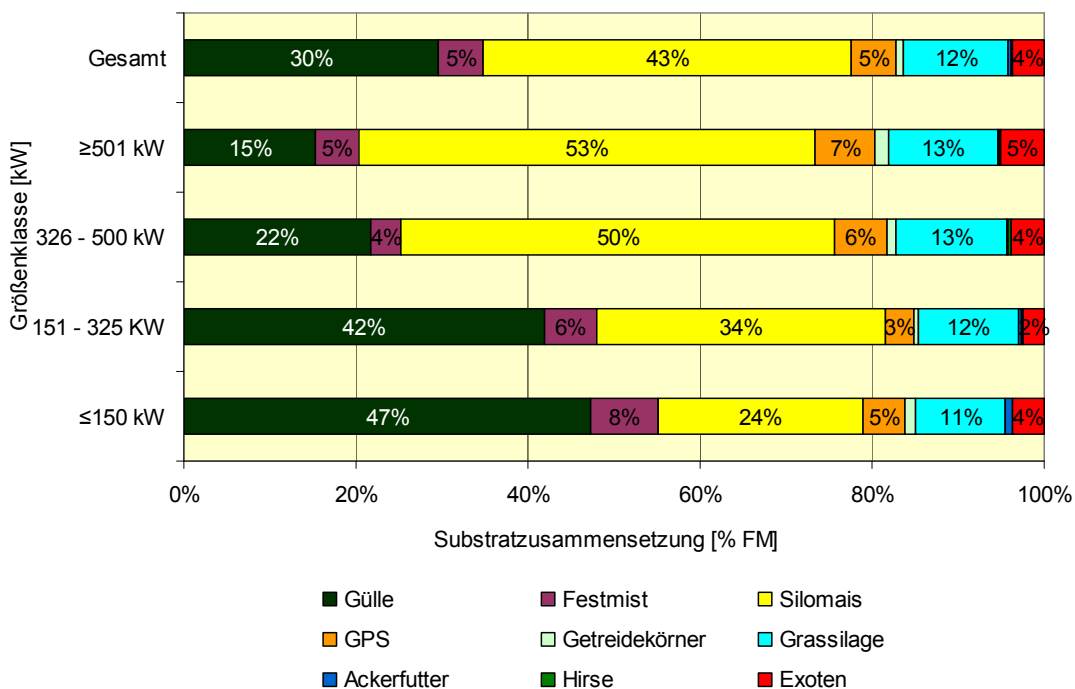
Abbildung 1: Substratmix (frischmassebezogen) von 81 befragten Biogasanlagen in Baden-Württemberg (Stenull et al., 2011).
