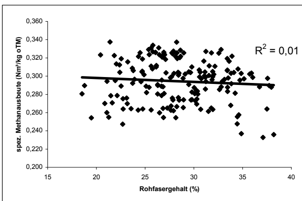
Abbildung 8: Zusammenhang zwischen Rohfasergehalt und spez. Methanertrag
