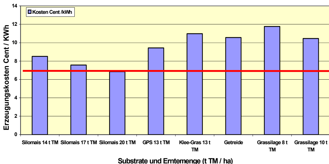
Abbildung 2: Erzeugungskosten der Biomasse je kWh Strom (Messner, 2009)
