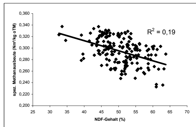
Abbildung 9: Zusammenhang zwischen NDF-Gehalt und spez. Methanertrag
